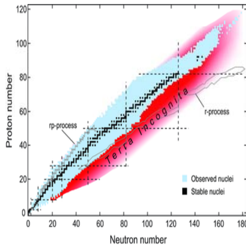
安定・不安定原子核の分布
