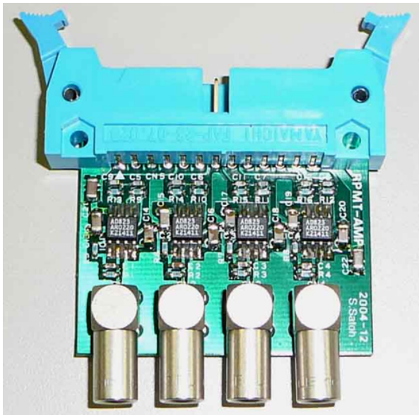
写真 8 RPMT_AMP 基板の外観図
