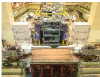
最終収束超伝導電磁石 (QCS)
