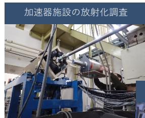
電磁石の放射化イメージング
