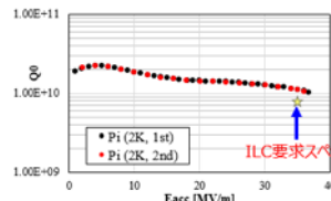
Large Grain 加速空洞の性能評価
