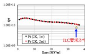
Large Grain 加速空洞の性能評価
