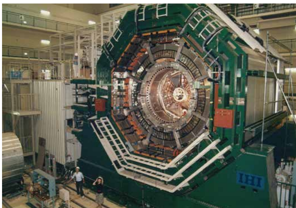
トパーズ測定器建設風景 (1980年代中頃)
