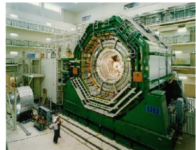
トパーズ(TOPAZ)測定器用タイムプロジェクトン・チェンバー(TPC)の組み込み
