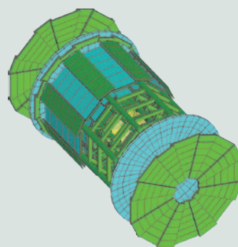
DAWN: 検出器や粒子の飛跡を高精度に描画するソフトウェア。図は ATLAS 実験の検出器
