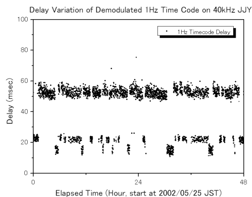
図 3. タイムコード復調時刻精度
