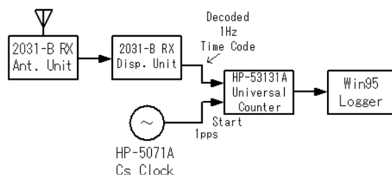
図 2. タイムコード復調時刻精度測定装置構成
