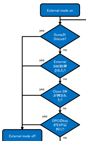
図 6 External mode が off になる条件
