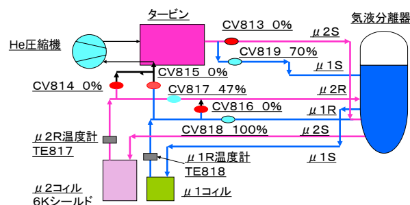
図4 シリーズ冷却回路
