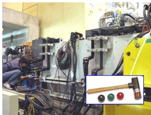
図 3 : モーダルインパルステスト試験風景。
