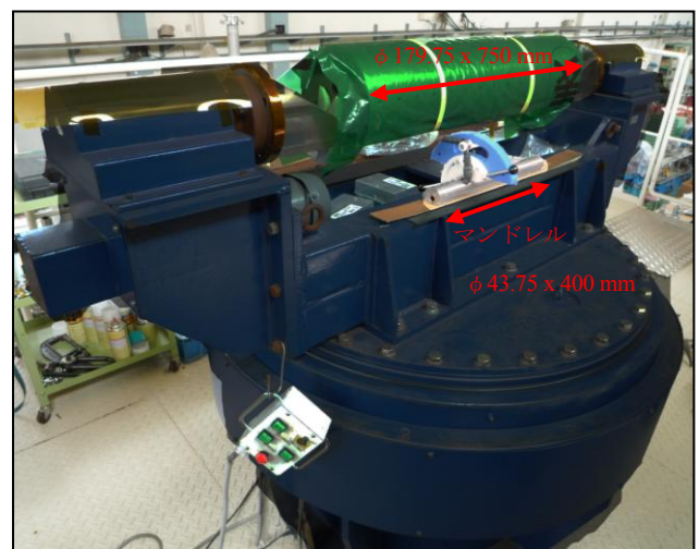
図 8-6 新旧巻き線機（マンドレル）の形状比較 (φ179.75x750mm : 2005 年 Super KEKB の R&D)
