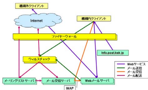
図 1 KEKmail 構成概略図
