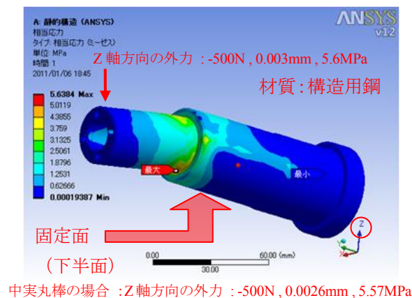
図 6-1 車軸貫通穴（ \phi 15\text{mm} ）の強度解析
