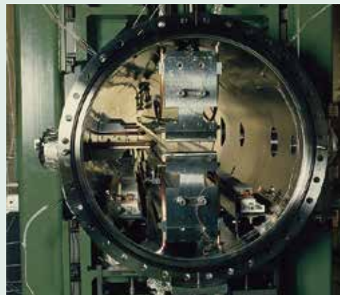
世界初の真空封止型アンジュレーター (AR-NE3)
