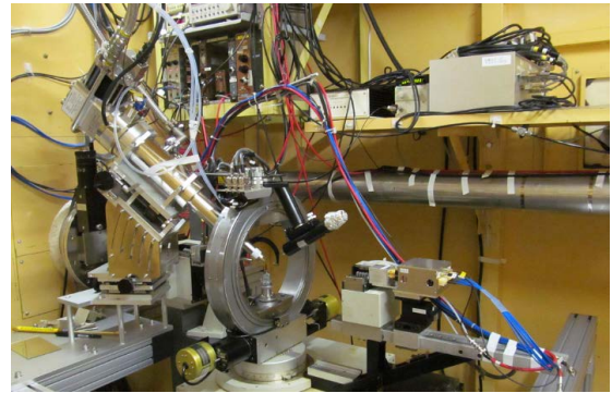
図 1 BL-14A で運用中の水平型四軸回折計と高計数率 APD 検出器 (写真右下, 20 アーム上に搭載)
