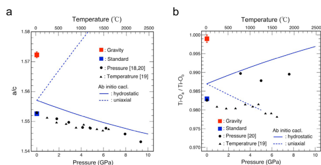
図2 超重力因果 \text{TiO}_2 ルチル単結晶 (赤■) の軸比 c/a (a) と \text{TiO}_6 八面体の結晶学的に非等価な2種類のTi-O距離の比率 ( \text{Ti-Oa}/\text{Ti-Ob} ratio) (b)。温度や圧力依存性と異なる独特の大きな構造変化を持った構造が得られる [1]。
