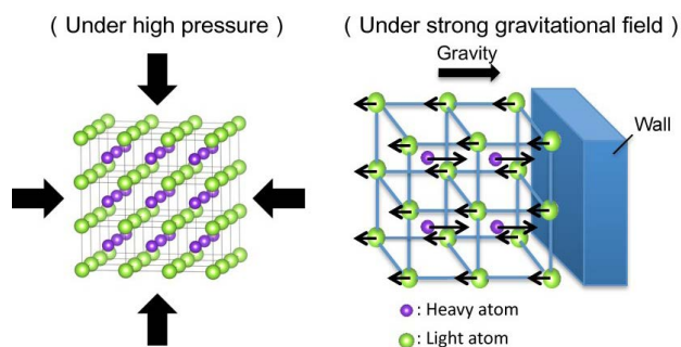
図1 静水圧印可と超重力印可では単結晶構成原子への効果が異なる。壁がある場合、軽い元素は浮力がかかり、一軸方向に元素の密度差等で原子の移動が起こる。温度急冷等を用いて、歪んだ構造を凍結できる [1]。
