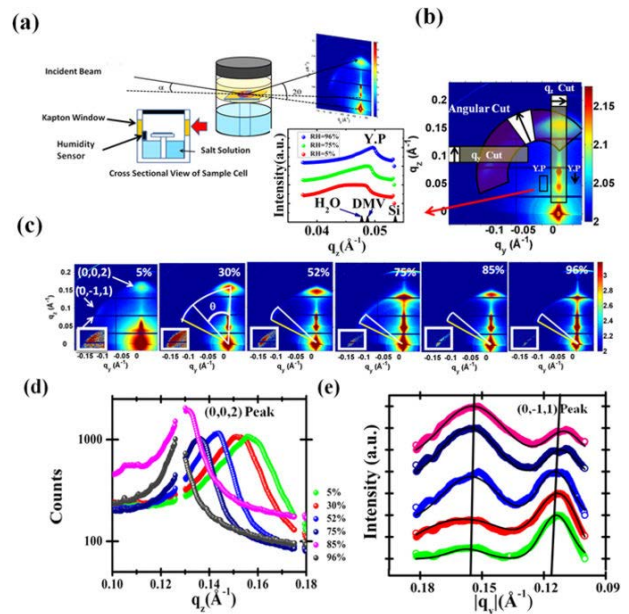
図 1 (a) ドデシル・メチルピオローゲン (DMV)-コロネンテトラカルボン酸カリウム塩 (CS) を用いた自己組織化ナノファイバーの斜入射 X 線小角散乱の相対湿度依存性測定の模式図。(b) 得られた回折像から波数依存性への変換。(c) 回折像の相対湿度依存性。(d) (e) 水平、垂直方向の回折強度プロファイルの相対湿度依存性。湿度によるファイバーの構造変化の様子を示している。
