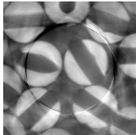
図2 X線位相ラミノグラフィーによるプラスチックビーズ(直径約3mm)の再構成画像
