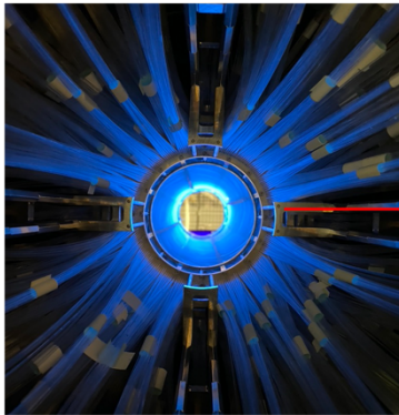
内側のファイバー検出器の写真
