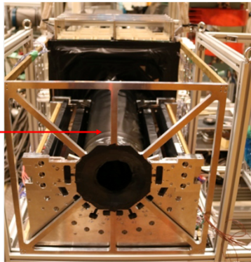
CATCH検出器の組み立て時の写真
