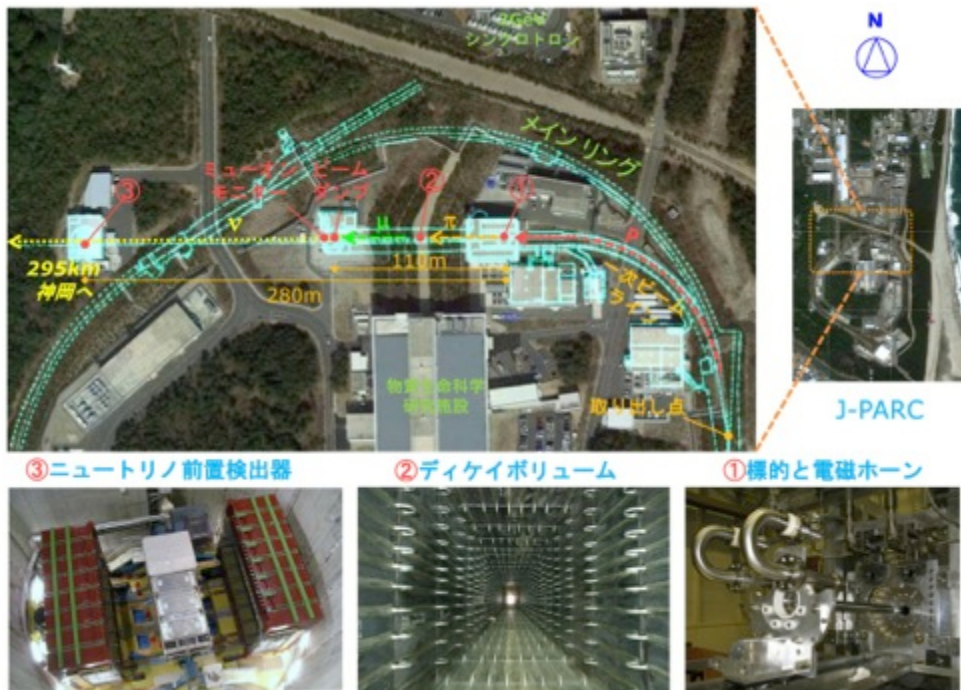
図 1 : T2K 実験の概要
