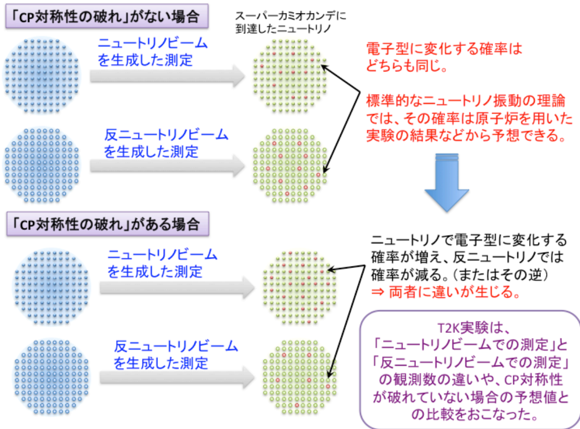
図 6 : T2K 実験で予想される「CP 対称性の破れの効果」
