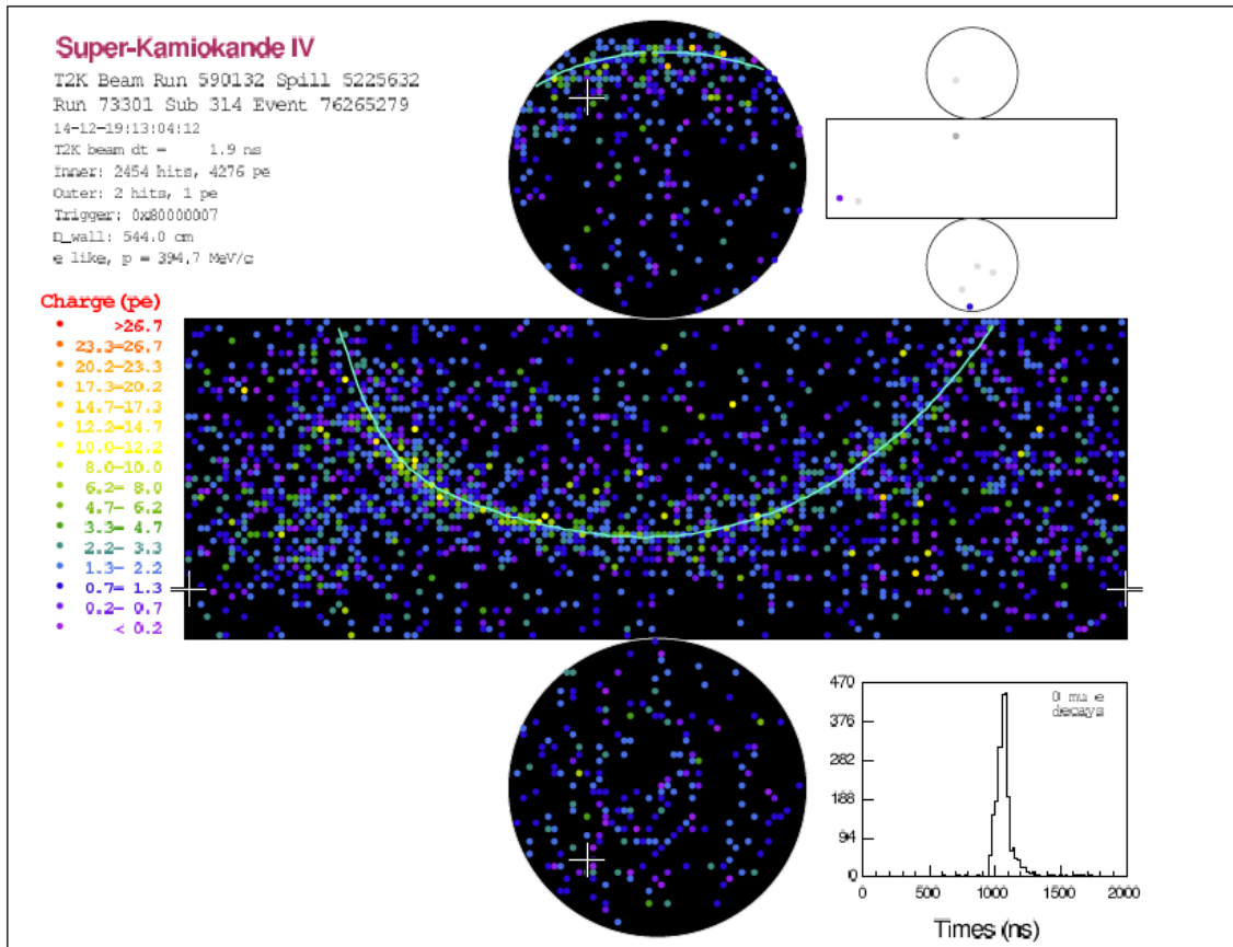
図 8 : スーパーカミオカンデで検出した J-PARC からの反ニュートリノビームに由来する反電子型ニュートリノ反応の事象
