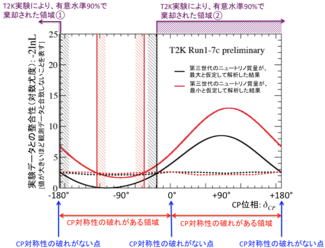
図 9 : T2K 実験から評価した CP 対称性の破れの大きさ
