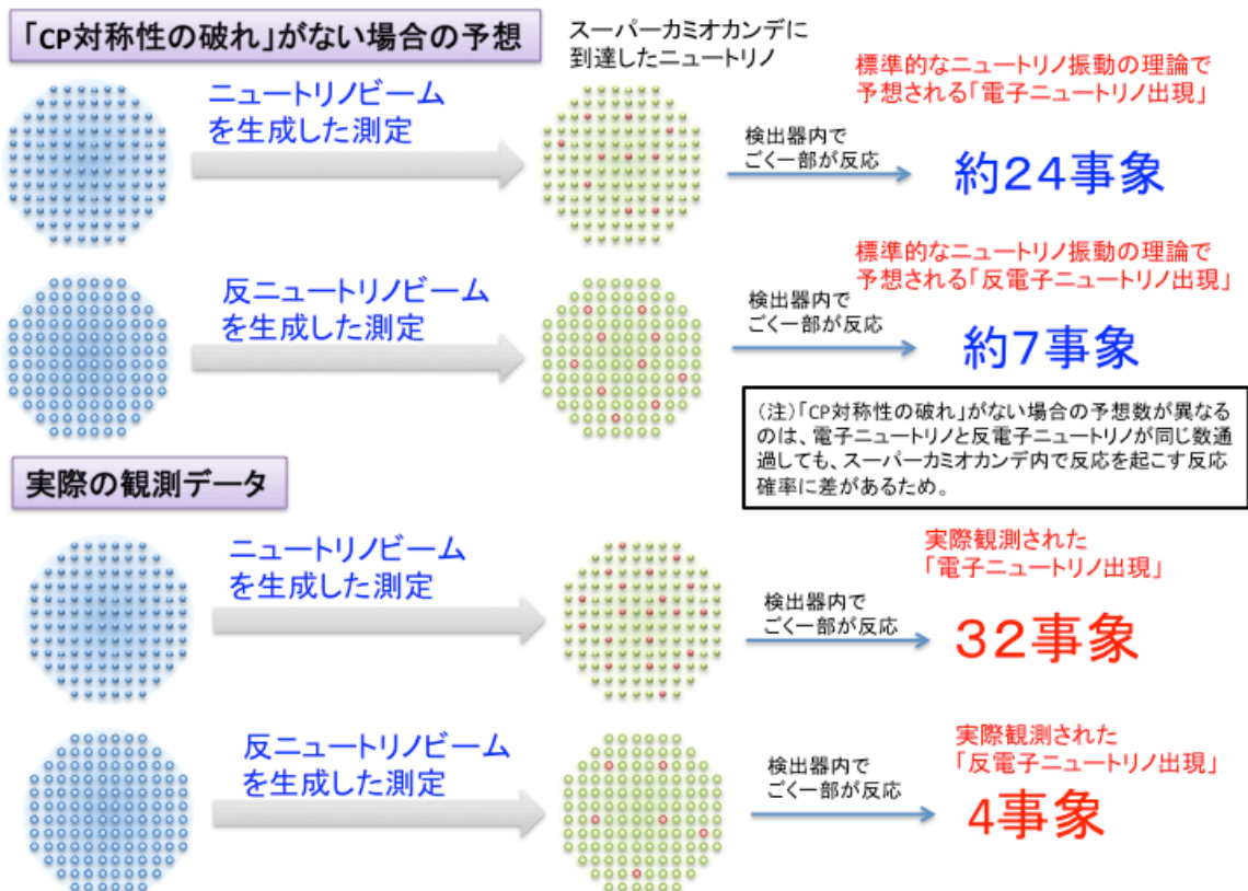
図 7 : T2K 実験での観測数と予想値の比較
