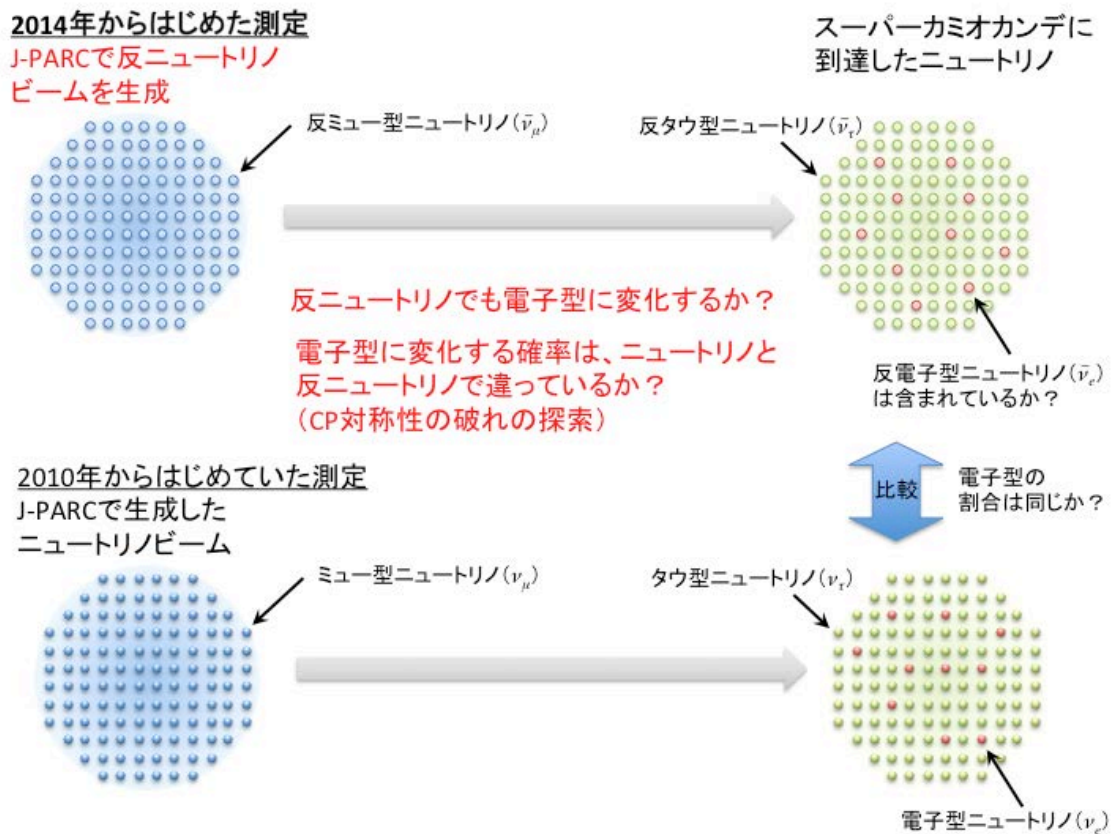
図 5 : ニュートリノ振動、反ニュートリノ振動の両方を測定できるT2K実験
