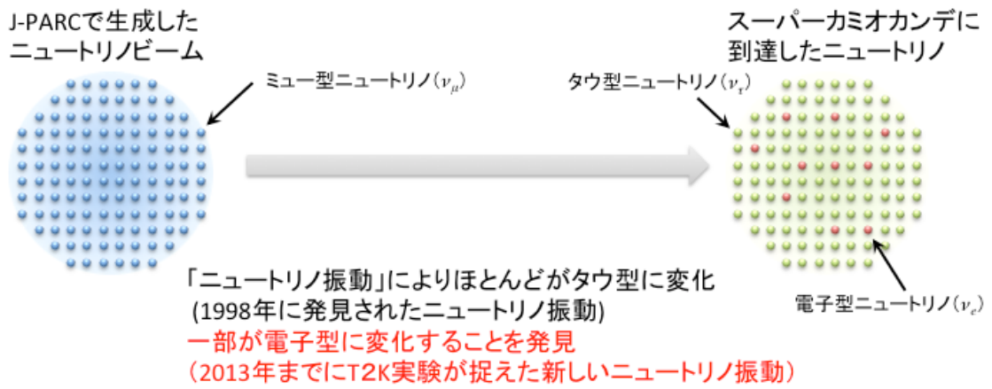
図 4 : 2013年にT2K実験が直接検出したミュー型から電子型へのニュートリノ振動 「電子型ニュートリノ出現」の模式図
