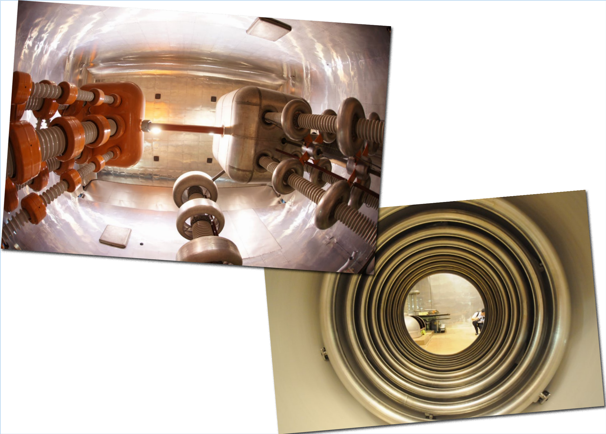
KEK PS 前段加速器（左） 下から見上げたコッククロフト＝ウォルトン型加速器（右） 前段加速器で使われた加速空洞
