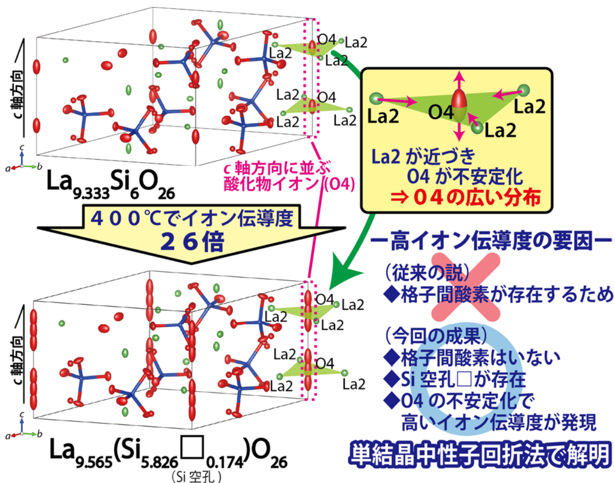
図 2：単結晶中性子回折法で明らかにしたアパタイト型酸化物イオン伝導体 La 9.333 Si 6 O 26 および La 9.565 (Si 5.826 □ 0.174 )O 26 の結晶構造と高いイオン伝導度発現の要因
