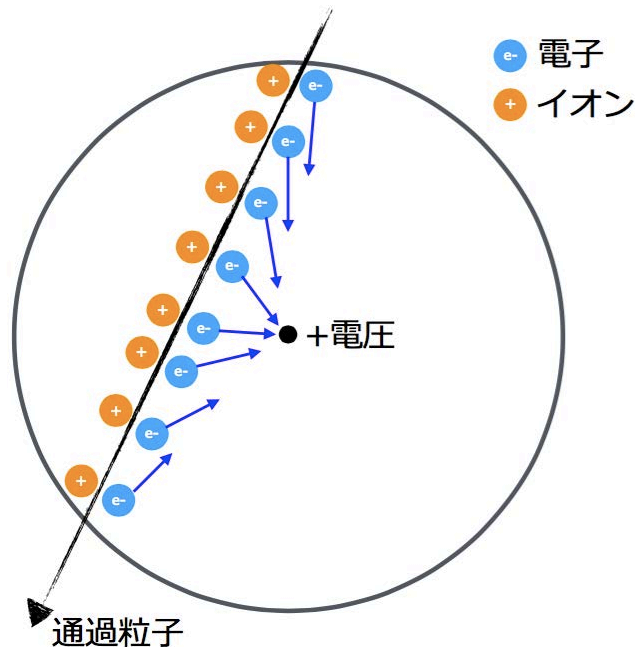
図 2.4 ガス検出器の基本的な動作原理
