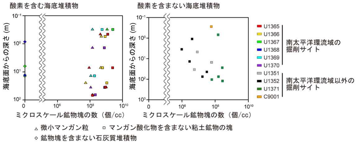
図3 海底堆積物試料 1 cc に含まれるミクروسケール鉱物塊の数の深度プロファイル。
