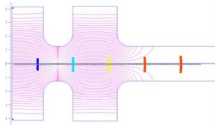
図 2 : 電気力線とビーム軌道
