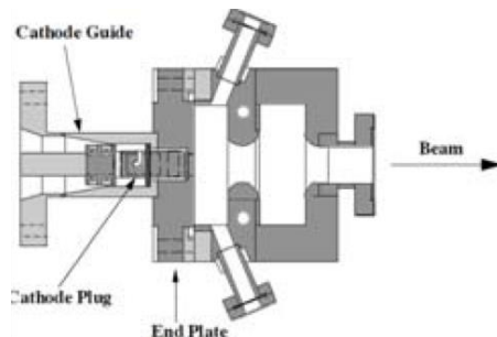
図 1 : 高周波電子銃
