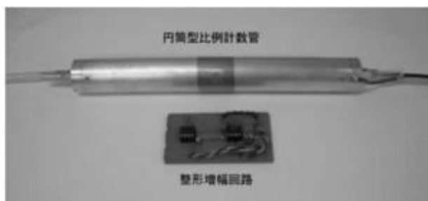
この演習で作成するワイヤーチェンバー (円筒形型比例係数管)と増幅回路
