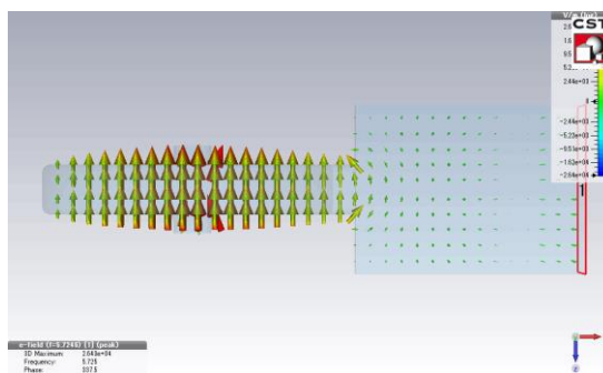
図5 : 電磁波シミュレーション
