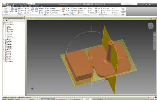
図4 : 3次元CAD
