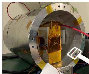
実習で作成した NMR 装置
