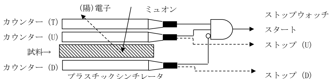
図 2 宇宙線版ミュオンスピン回転観測装置
