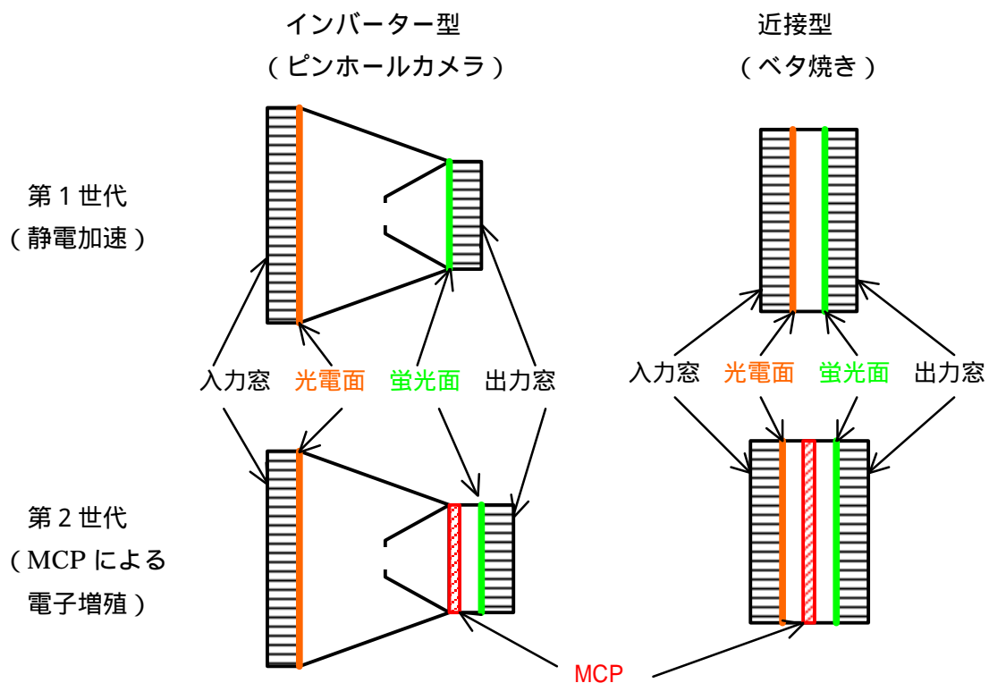
図 2 - 1 : イメージンテンシファイアの分類
