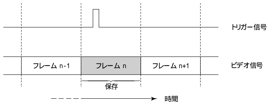
図 3-1 : パソコンに入力されるビデオ信号とトリガー信
