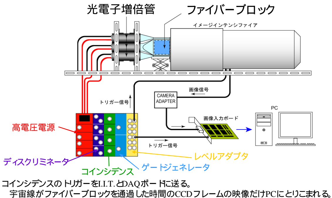
図 1-3 実験装置全景
