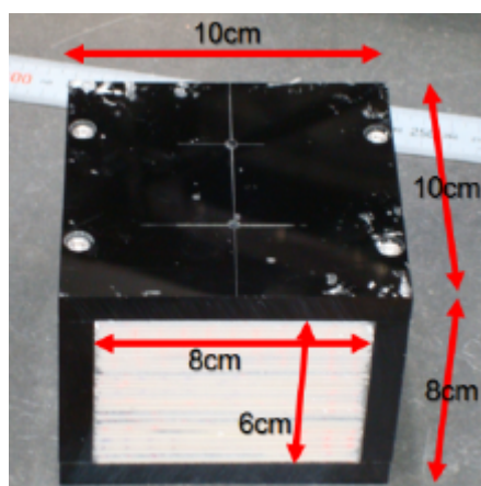
図 1-2 KEK サマーチャレンジ 2007 で製作した SciFi ブロック
