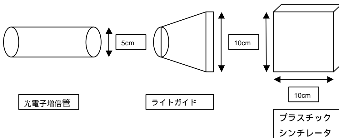
図 4-2 トリガーカウンター。ライトガイドとプラスチックシンチレータはオプティカルセメントで接着するが、光電子増倍管とライトガイドはオプティカルグリースで接触させるだけにする。
