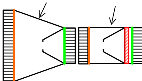
図2 - 3 : イメージンテンスファイアチェーン (複数のイメージンテンスファイアをつないだもの)
