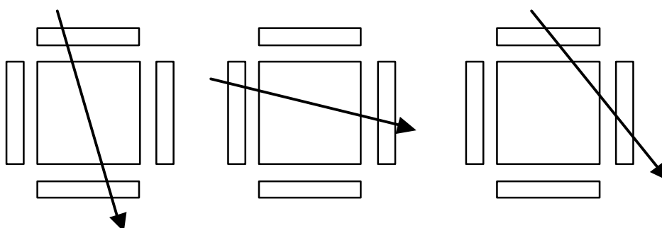
図 4-1 検出器の正面図。ファイバーブロック(中央の正方形)の周囲4面をプラスチックシンチレータで囲み、4面中2面を宇宙線(矢印)が通過した時にデータを取得するようにセッティングする。
