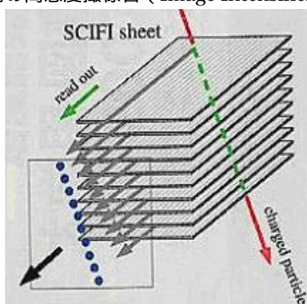
図 1-1 SciFi ブロックによる荷電粒子の観測
