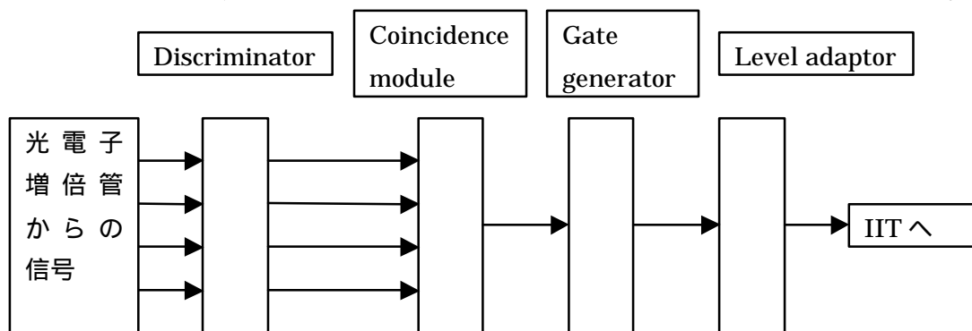
図 4-3 電子回路モジュール類の結線
