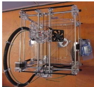
図4：3次元造型機
