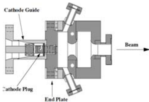
図1：高周波電子銃
