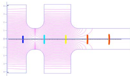
図2：電気力線とビーム
