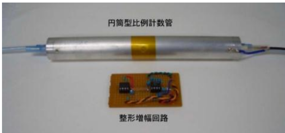
この演習で作るワイヤーチェンバー（円筒型比例計数管）と増幅回路
