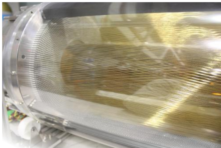
ドリフトチェンバーの例：東北大電子光理学研究センターで行っている NKS2 実験で使用
