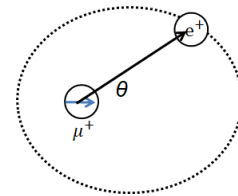
図1 b 崩壊陽電子の放出角分布
