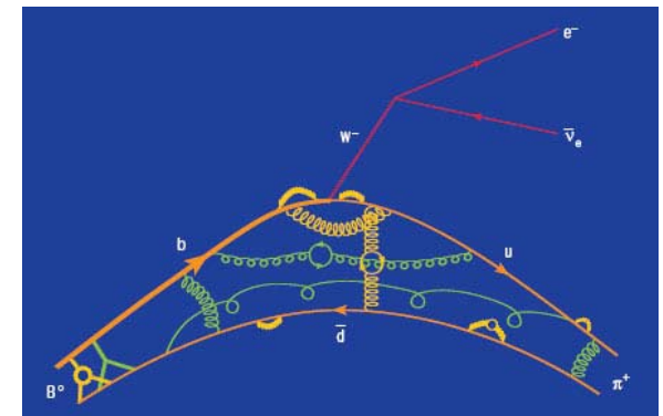
B中間子崩壊に寄与するダイアグラムの一例
