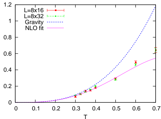
ブラックストリングの 内部エネルギーと圧力の差
